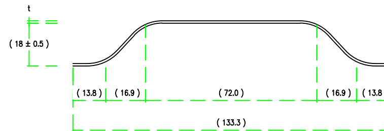
山谷部詳細寸法
