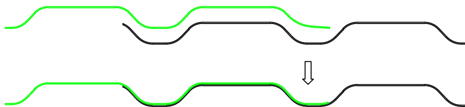
葺き合せ納り参考図
