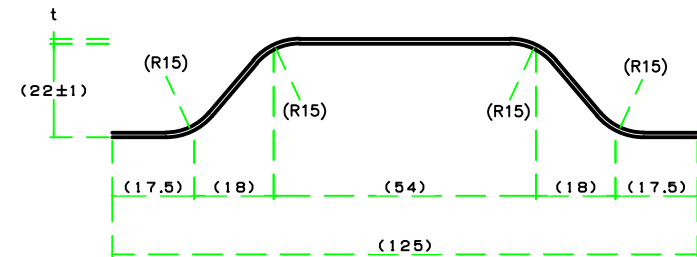
山谷部詳細寸法
