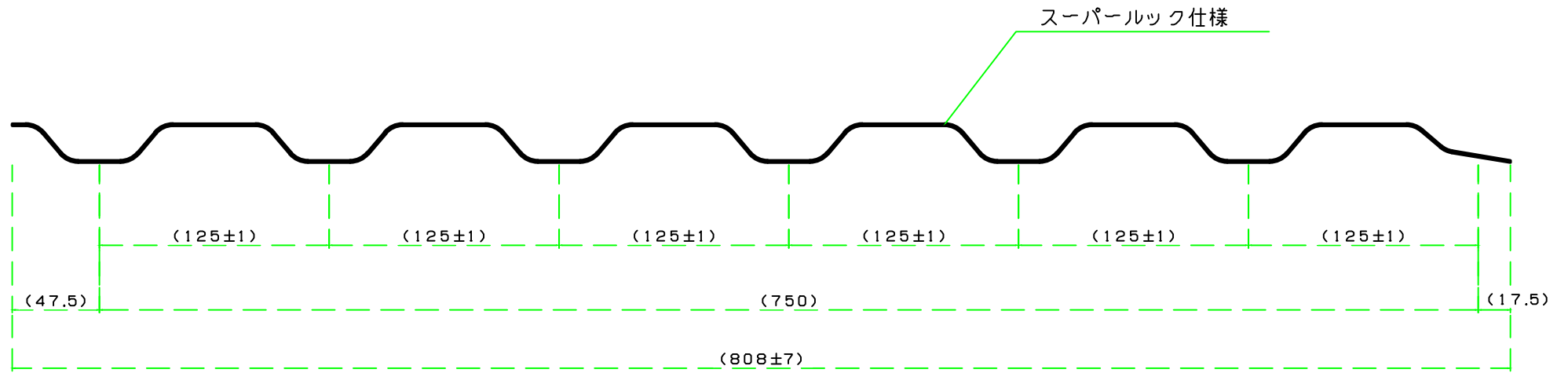
葺き合せ納り参考図
